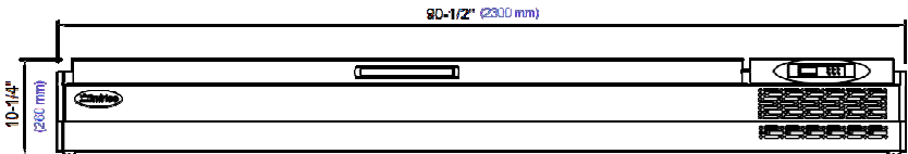
ELEVATION
